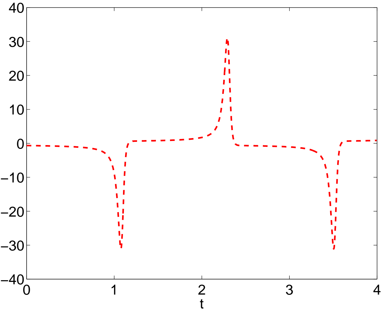
Van der Pol Gleichung, \mu = 20 , Ableitung y'(t)
