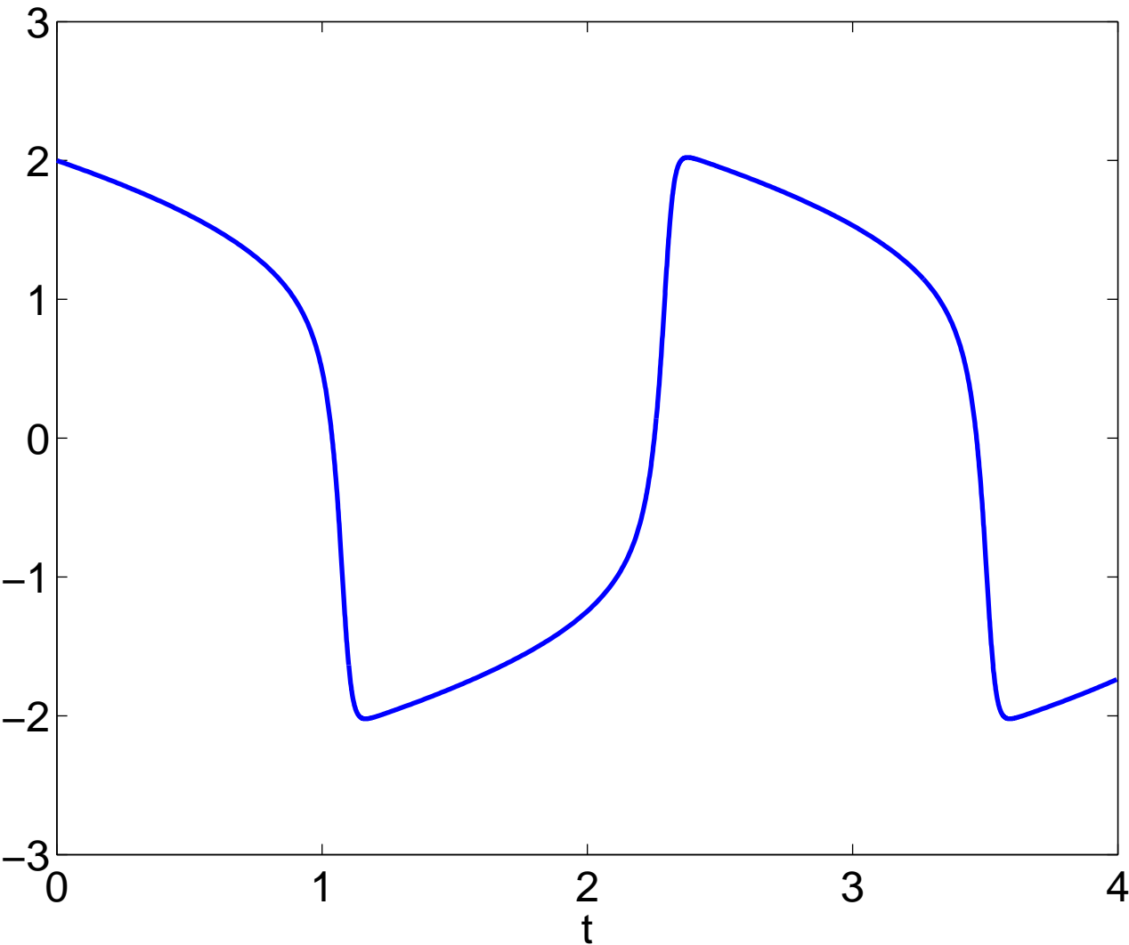
Van der Pol Gleichung, \mu = 20 , Lsg y(t)
